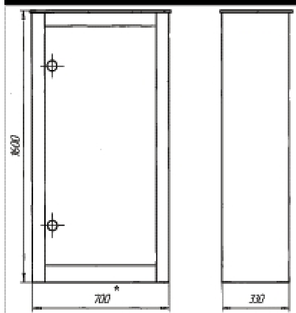
Рис. 6.1. Структура шкафов ШРС-11 и ШРС-1
